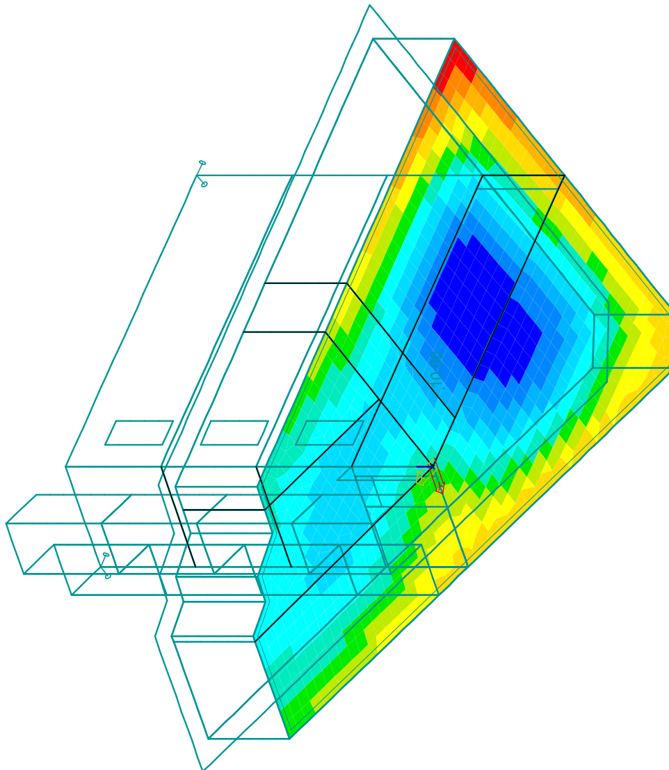
Contactspanning - max sigmz - FEM Combi : 1/2
